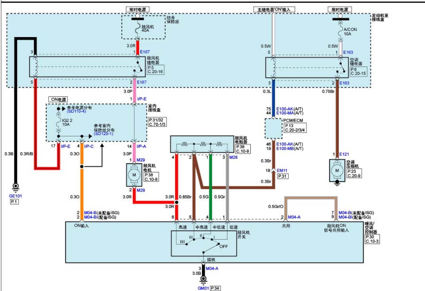
空调控制系统(1)
